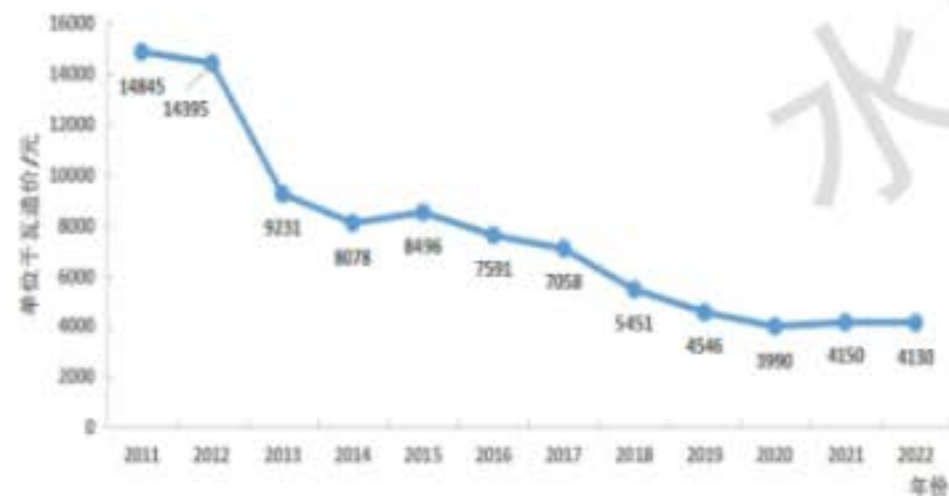
2011—2022年光伏发电项目单位千瓦造价指标变化趋势
