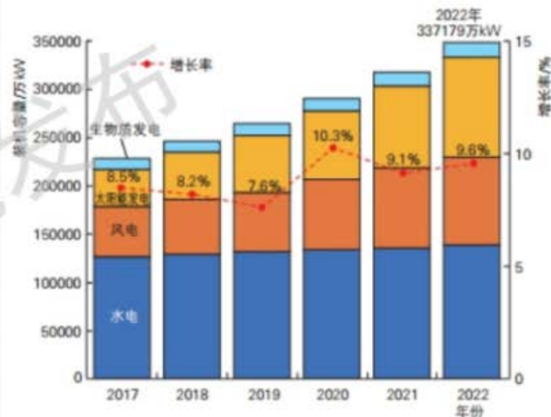
全球可再生能源发电累计装机容量和增长率 (2017—2022年)
