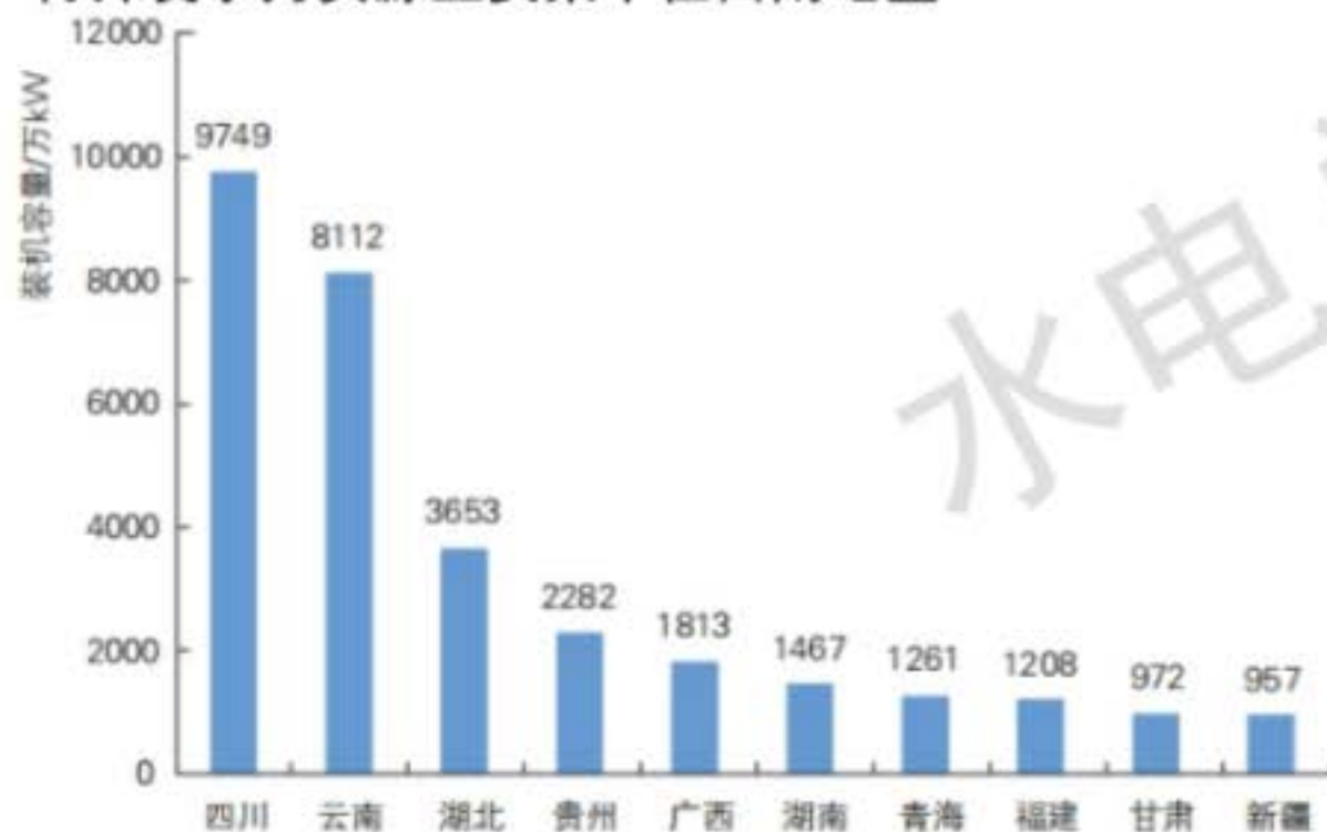
主要省份常规水电装机容量
